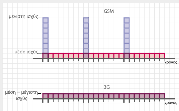
Σχήμα 8: Επίπεδα μέσης ισχύος στα τυπικά συστήματα κινητών επικοινωνιών
