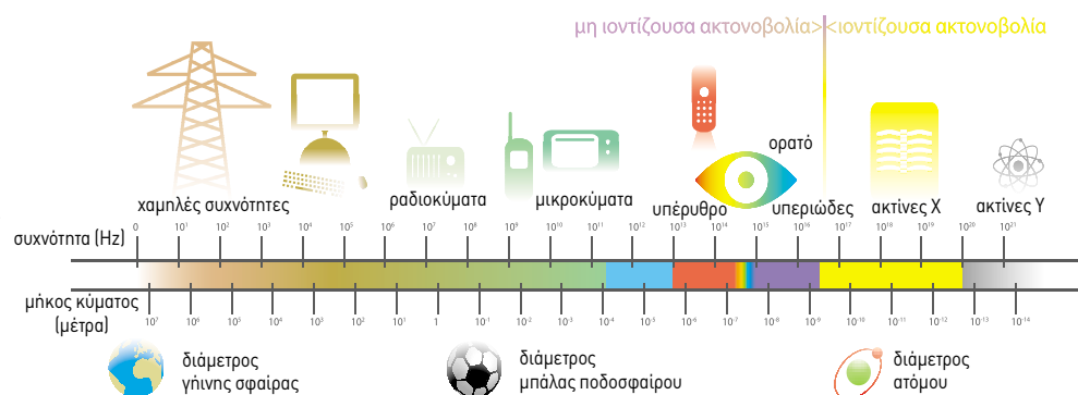
Σχήμα 1: Ηλεκτρομαγνητικό Φάσμα
